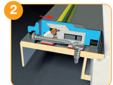
2 Mise en contact des lames avec le conducteur vert jaune par vissage
