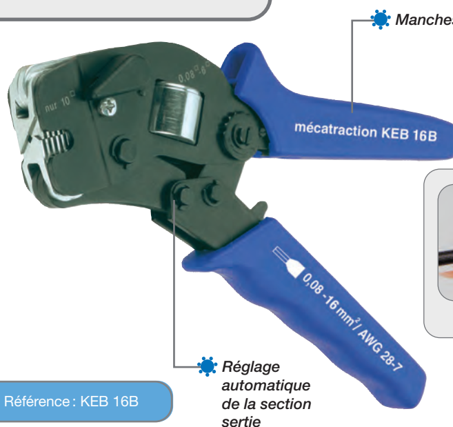
Sertissage latéral
